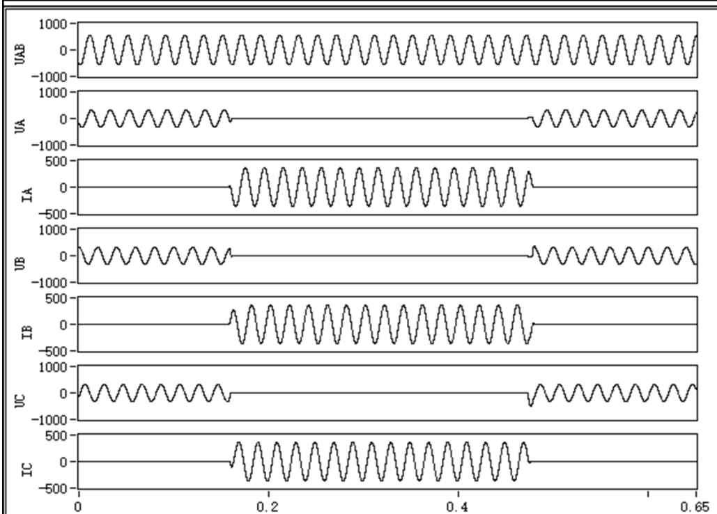
试验示波图
