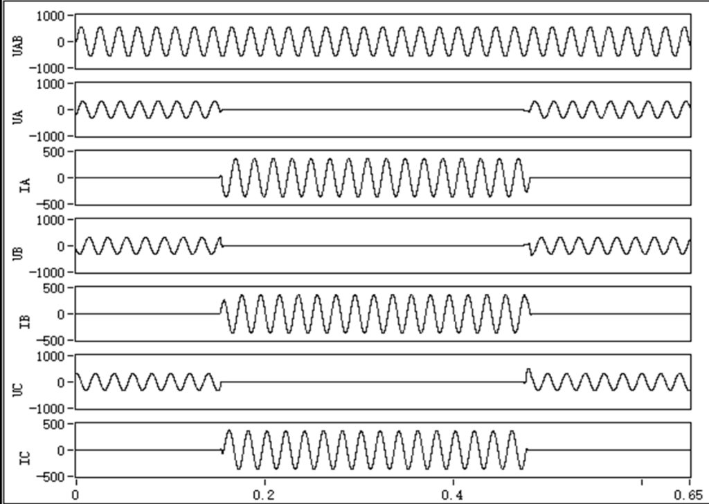
试验示波图
